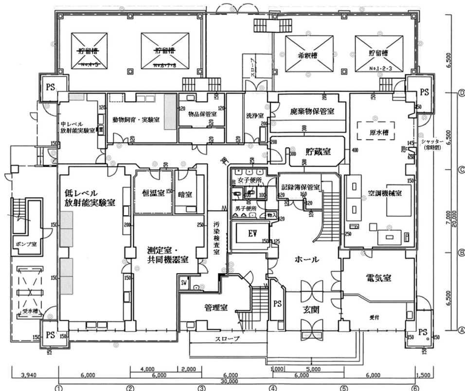
1階平面図
